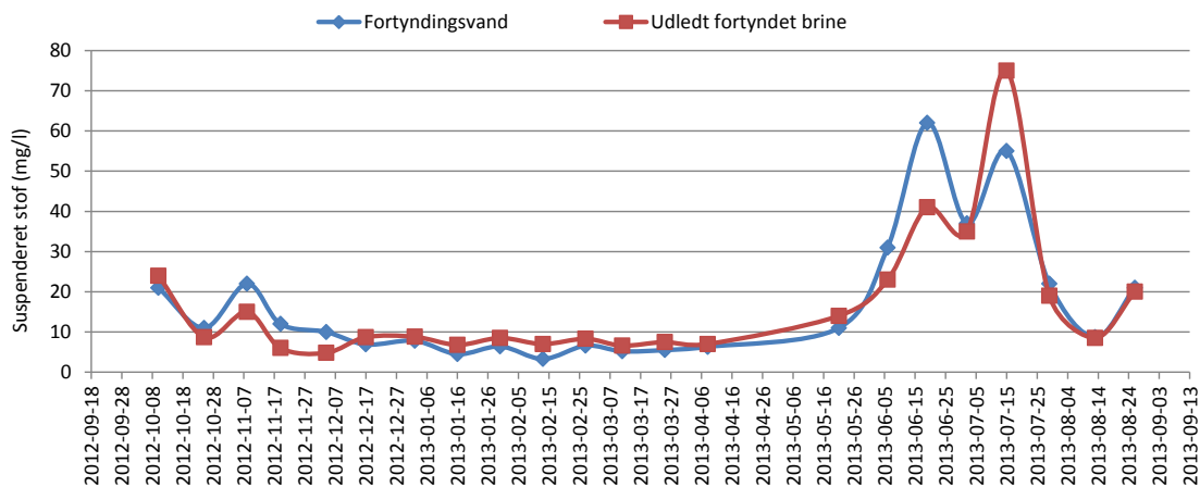
Figur 1 Suspenderet stof i fortyndingsvand fra Hjarbæk Fjord og udledt fortyndet brine
